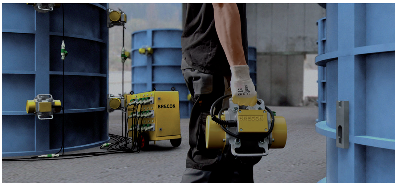
Быстросъемный вибратор Slim2 как часть вибрационной системы
