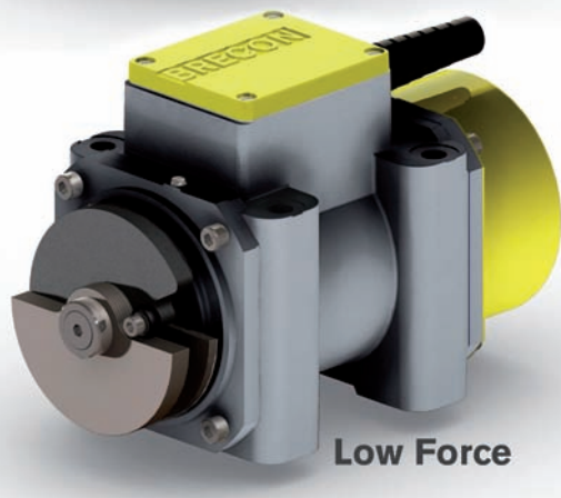
El motovibrador Brecon 2en1 posee dos curvas características diferentes dependiendo del sentido de la rotación.
