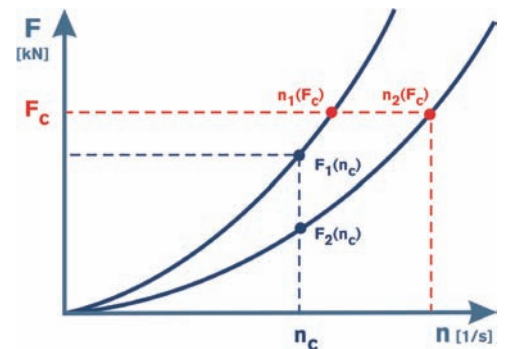
Los motovibradores Brecon 2en1 permiten el ser operados con dos curvas características diferentes.
