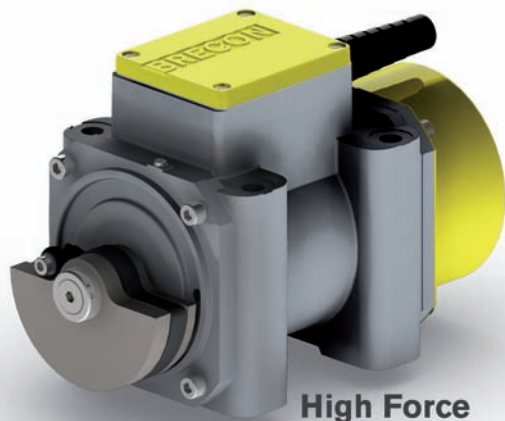
Una compactación en dos pasos con motovibradores Brecon 2en1 ofrece ventajas para productos con una armadura tupida.
