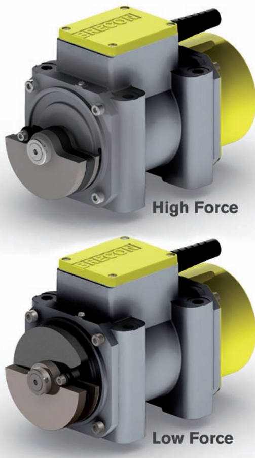
Fig. 3: Vibratore Brecon 2in1: in base al senso di rotazione si possono ottenere 2 curve caratteristiche diverse
