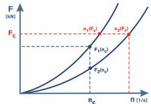
Fig. 2: I vibratori Brecon 2in1 possono essere utilizzati su 2 curve caratteristiche
