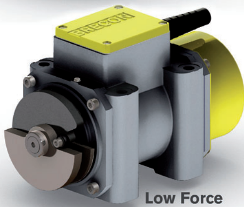
Вибратор Brecon 2-в-1: независимо от направления вращения работа проводится на двух различных кривых
