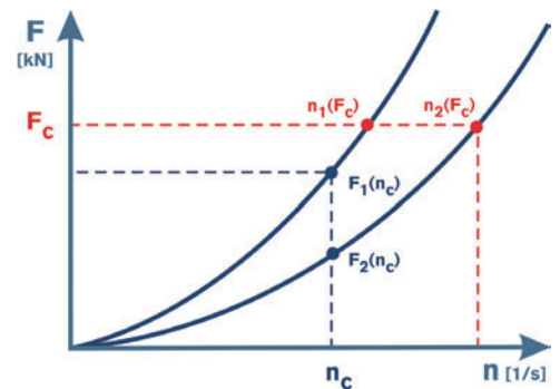
Вибраторы Brecon 2-в-1 позволяют работать на двух кривых
