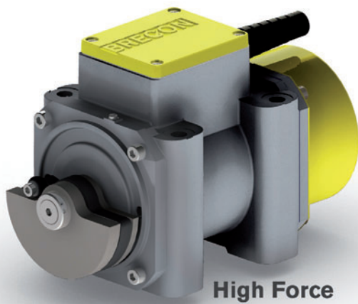
При высоком коэффициенте армирования двухэтапное уплотнение бетона при помощи вибратора Brecon 2-в-1 выявляет заметные преимущества
